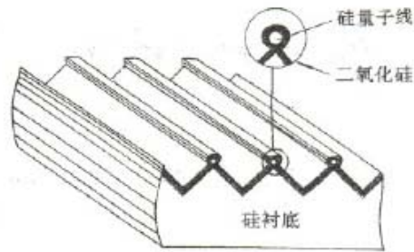
图 1 硅量子线阵列结构示意图
